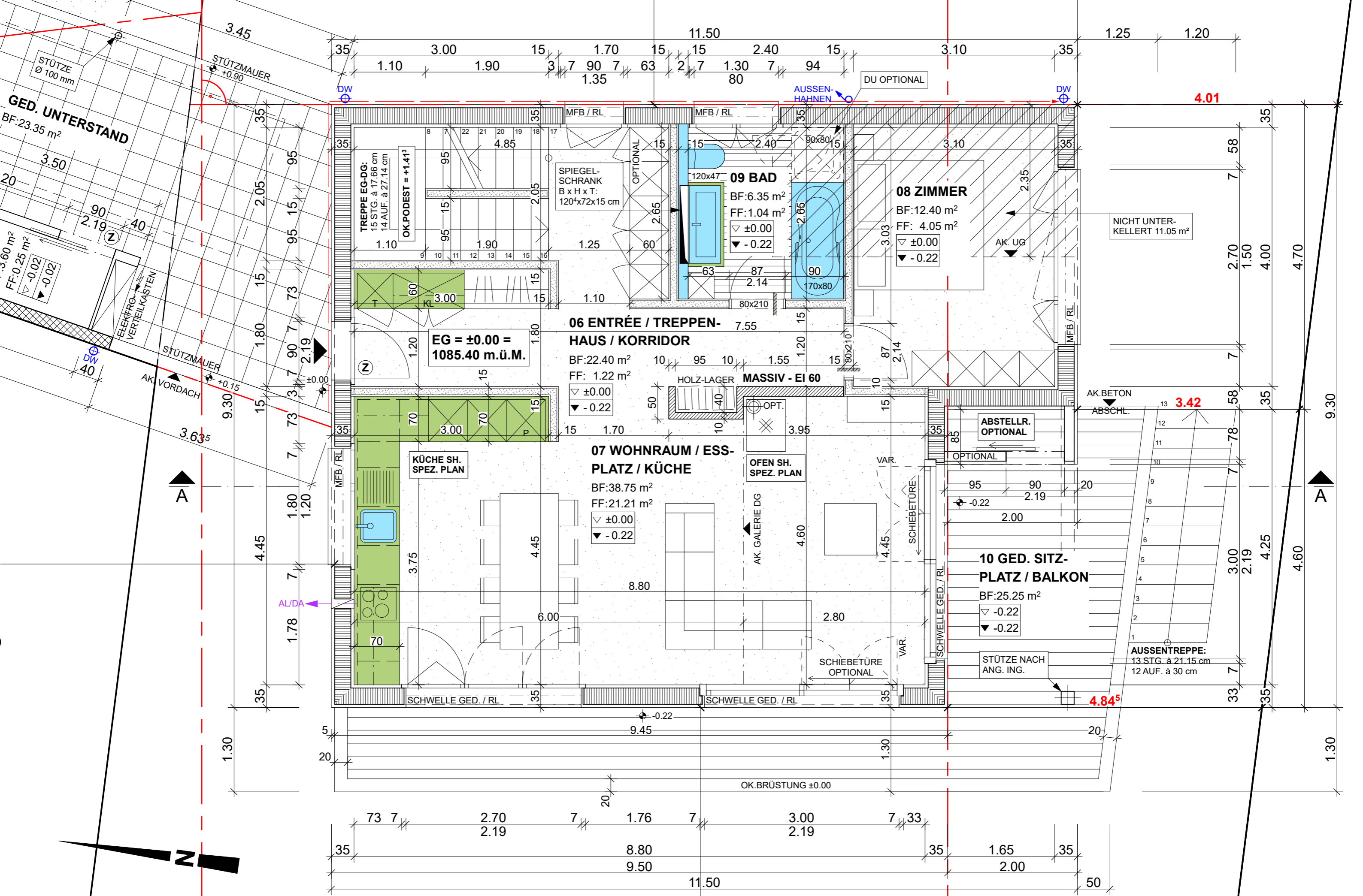
ERDGESCHOSS 1:50 HAUS A
